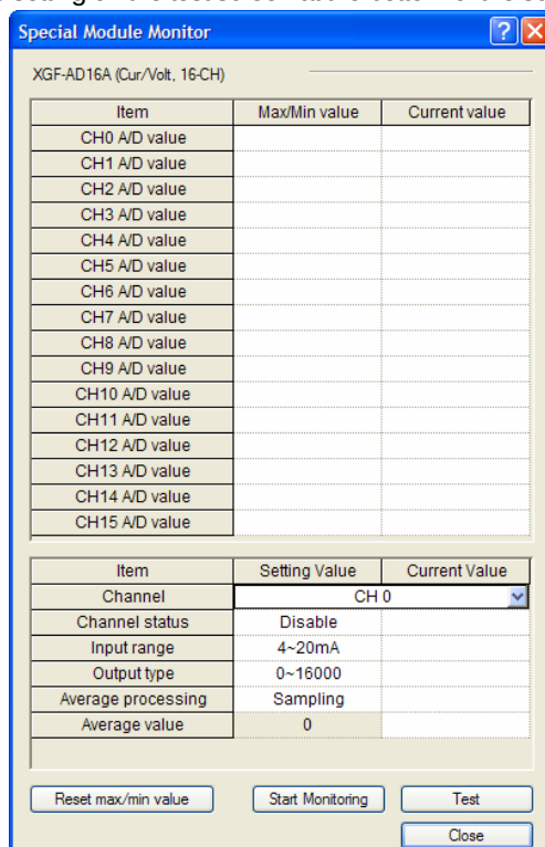
[Fig. 5. 3] [Special Module Monitoring] screen
