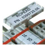
PEAD + RCPEAD-TT
