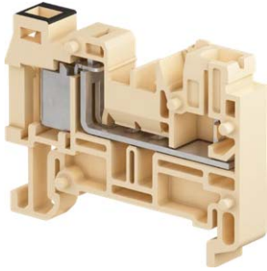
D2.5/7.ADO-CPE.NF1
