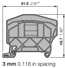
CS-R2
