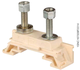
HD16/14.FF5.21
