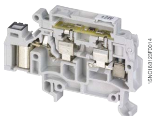
D4/8.SF.I.ADO
