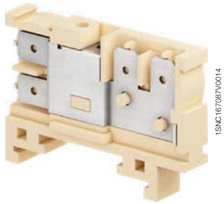
HD6/8.2G.2G.2
